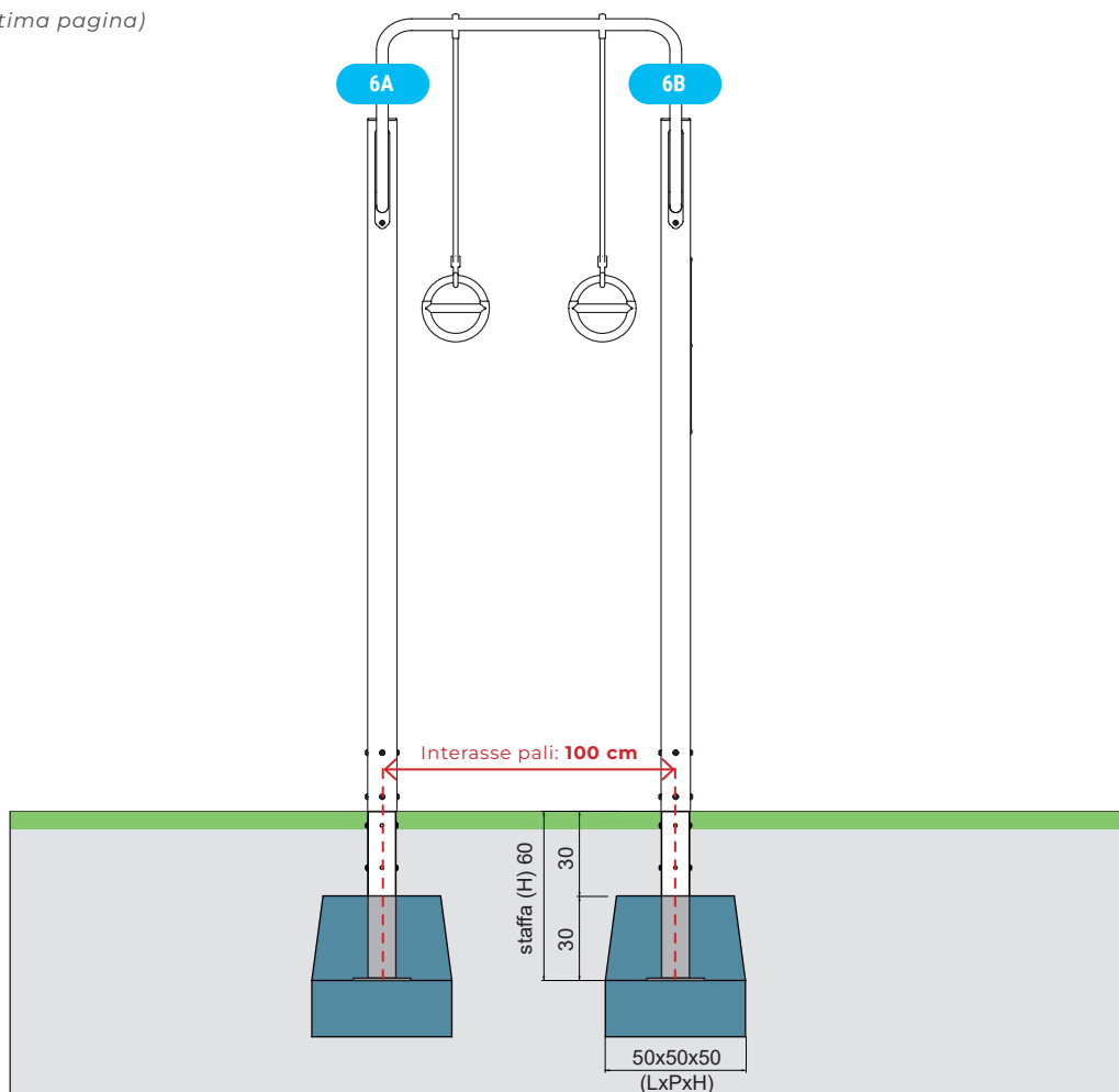
Dimensioni minime consigliate per plinti di fondazione.
