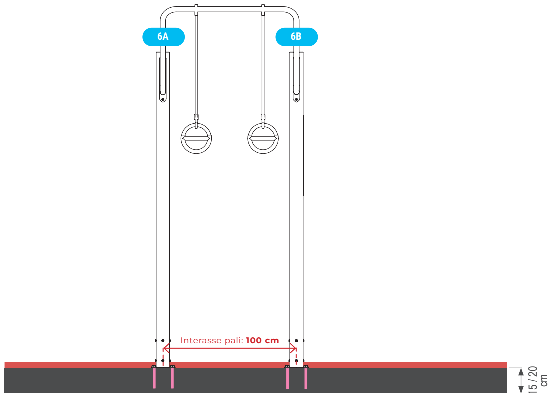
Altezza minima consigliata per piattaforma.
