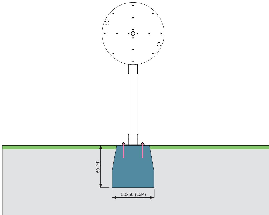
Dimensioni minime consigliate per plinti di fondazione.
